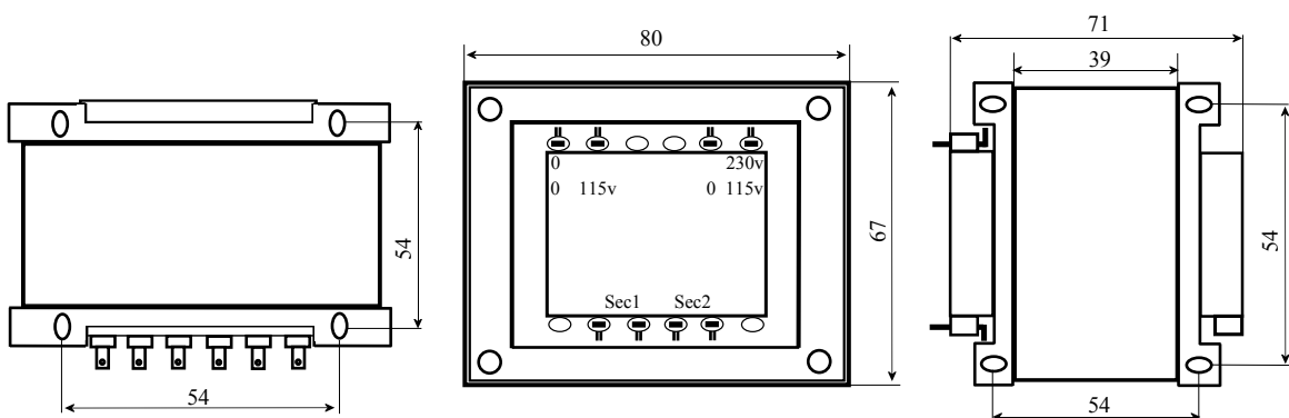
75VA
