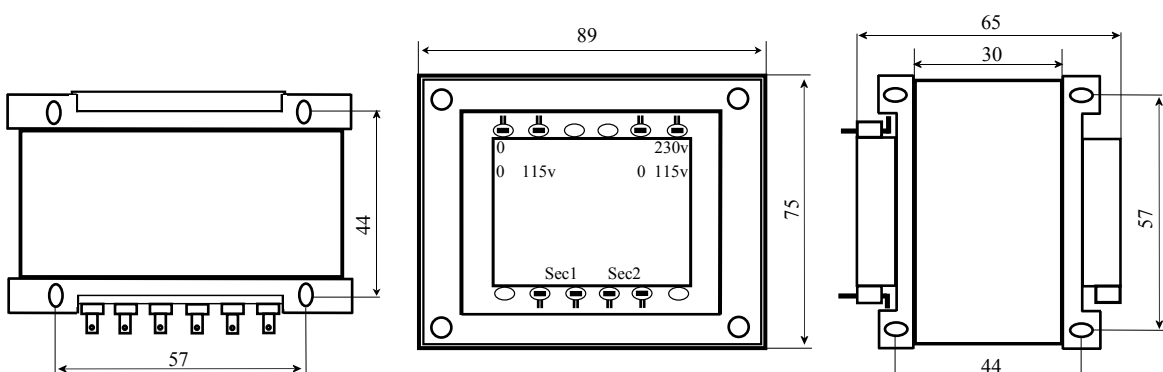
100VA
